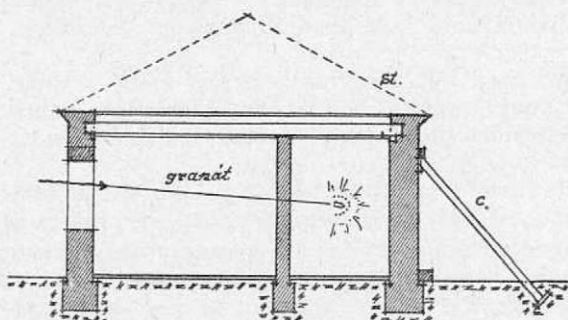
Náčrt 24.
