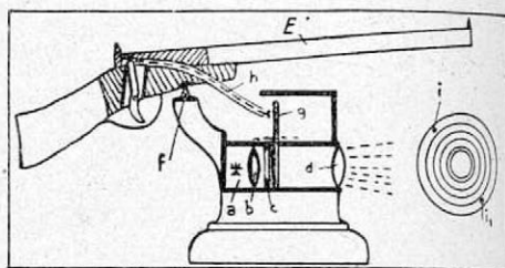
Obr. 2. Schematické znázornění střeleckého přístroje. Obr. 3. Kruhový terč.
