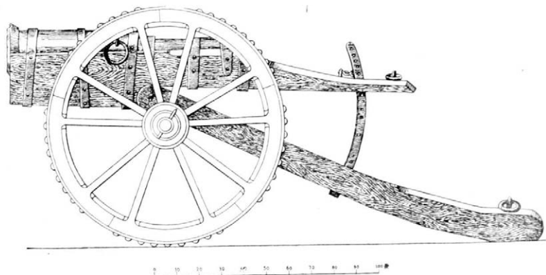
Obr. 13. Husitská houfnice z XV. století.
